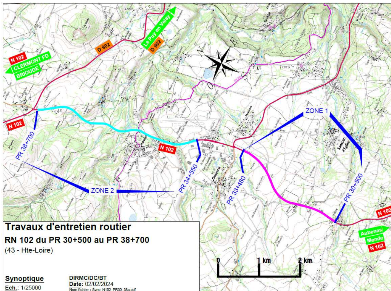
Plan de situation des travaux
