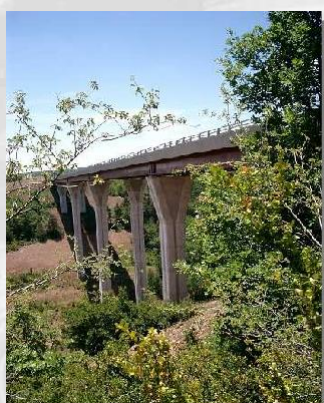
A75 - PR 212+000 : Viaduc de la Garrigue
