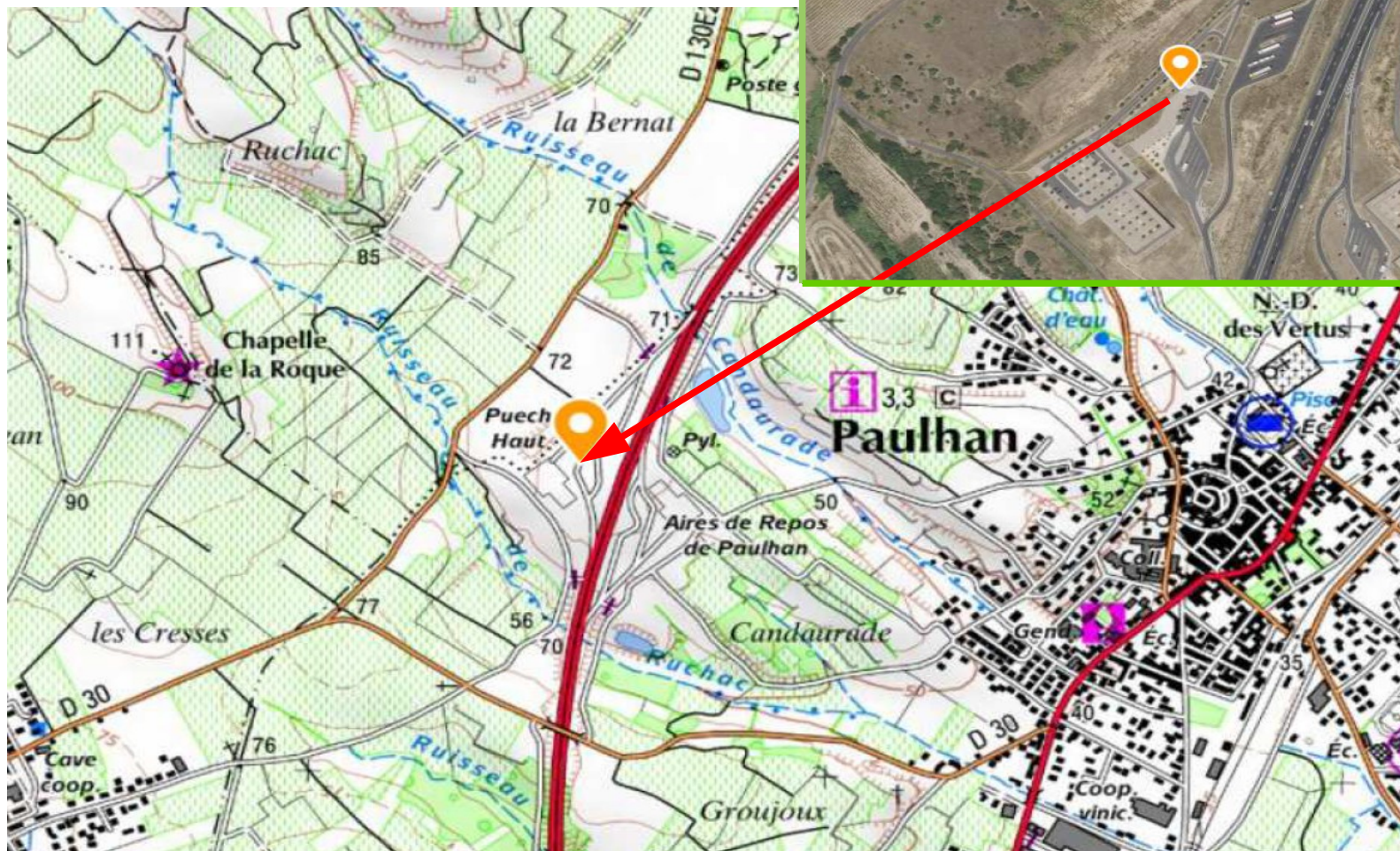
AIRE DE PAULHAN - Autoroute A75 – PR 303 Sens NORD→ SUD
